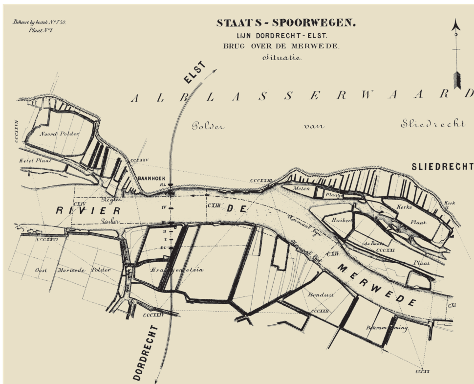
4.9 Bestektekening van de spoorbrug over de Merwede bij Baanhoek onder Sliedrecht.
