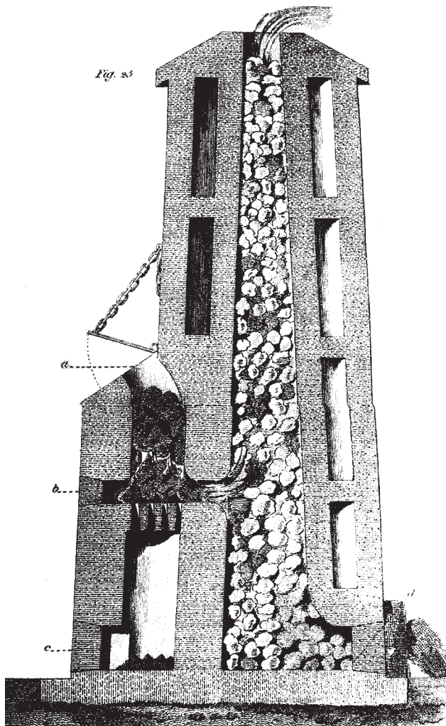
Afb. 4.4. De Rumford-kalkoven. Tegen het einde van de 18e eeuw was er een sterke toename te zien van de behoefte aan ongebluste kalk. De ovens waarin de kalksteen werd verhit, werkten langzaam en verbruikten veel hout als brandstof. Rumford ontwierp een nieuwe efficiëntere oven waarbij de verbrandingsschacht voor de kalksteen gescheiden werd van de brandstof. In het midden is er een constant vuur en bovenaan wordt de hoeveelheid kalksteen aangevuld.
