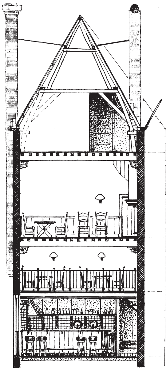
Langsdoorsnede van de 'De Pauw' na de restauratie.
